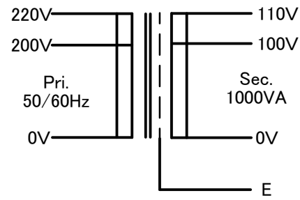
結線図
